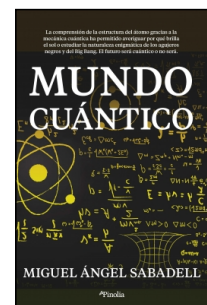
Mundo cuántico
