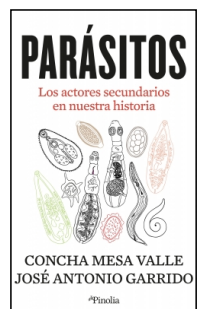
Parásitos
