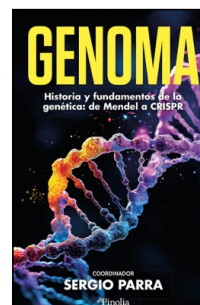
Genoma
