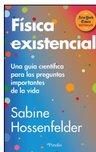
Física existencial
