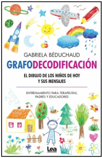
Grafodecodificación
